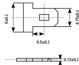
Conectori T1 (F1)
